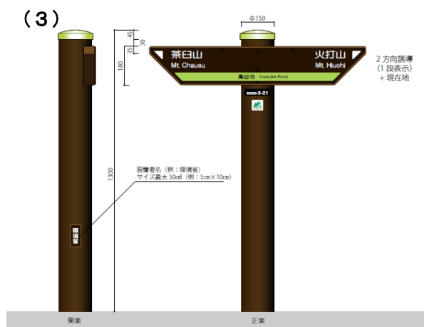
腕木タイプの誘導標識の標準デザイン
