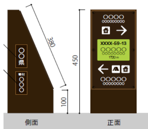
単柱（低）タイプの誘導標識の標準デザイン
